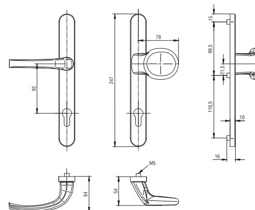
Klamka drzwiowa z gałką / Knopfgrünitur
