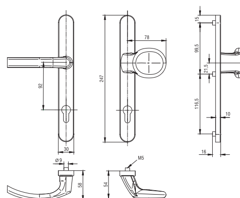
Klamka drzwiowa z gałką / Knopfgriffgarnitur
