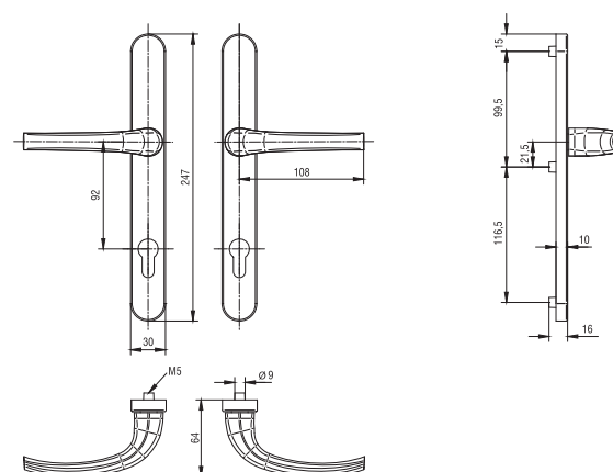
Klamka drzwiowa / Drückergarnitur
