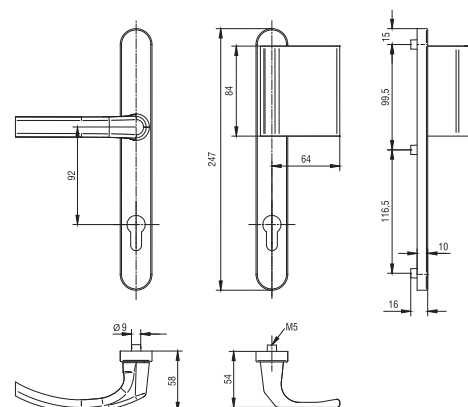
Klamka drzwiowa z pochwytem typu L / Stossgriffgarnitur
