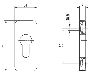
Szyld wkładki patentowej prostokątny
