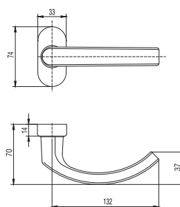
Klamka drzwiowa dzielona z szyldem owalnym
