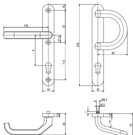
Klamka drzwiowa z pochwytem typu V
