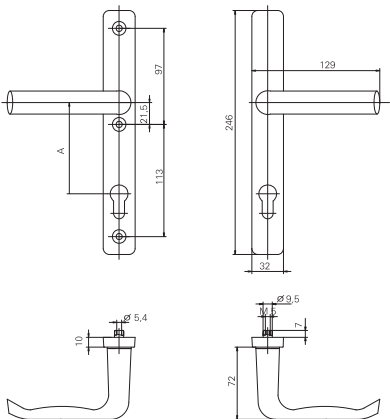
Klamka drzwiowa wysoka bez wspomagania, z jednostronnym lub dwustronnym mechanizmem sprężynowym
