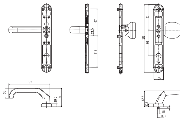
Klamka drzwiowa z galką
