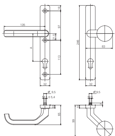
Klamka drzwiowa z gąlką stałą lub obrotową
