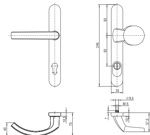
Klamka drzwiowa z pochwytem P
