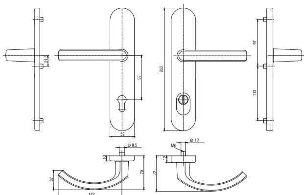
Klamka drzwiowa
