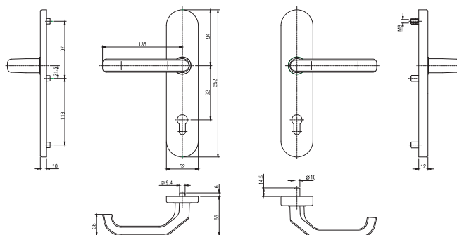
Klamka drzwiowa
