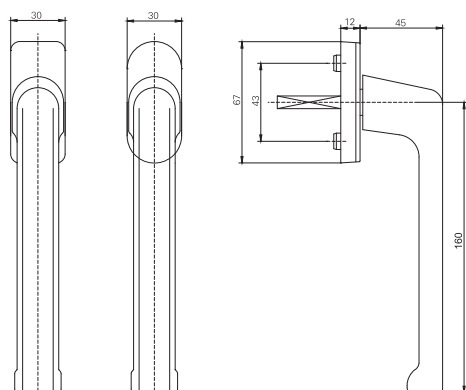
Klamka do drzwi przesuwnych z kluczykiem
