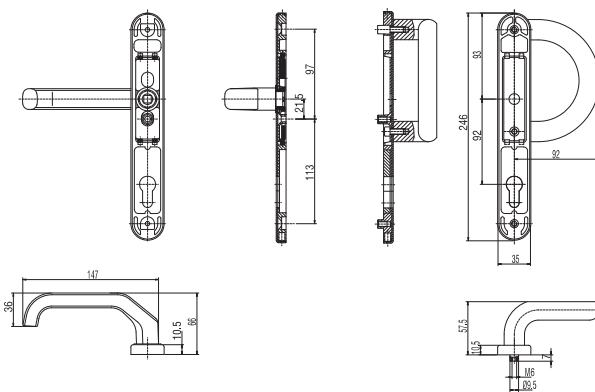
Klamka drzwiowa z pochwytem
