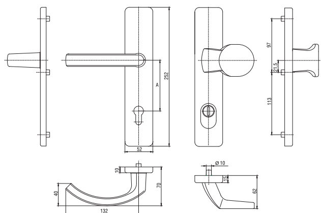
Klamka drzwiowa z gałką
