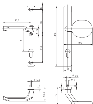
Klamka drzwiowa z gąlką stałą lub obrotową
