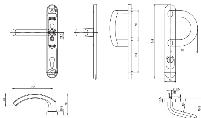
Klamka drzwiowa z pochwytem P
