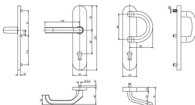
Klamka drzwiowa z pochwytem typu P
