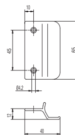
Uchwyt balkonowy z odsadzeniem
