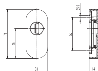
Szyld wkładki patentowej z antywłamaniową ochroną
