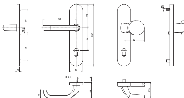
Klamka drzwiowa z gałką
