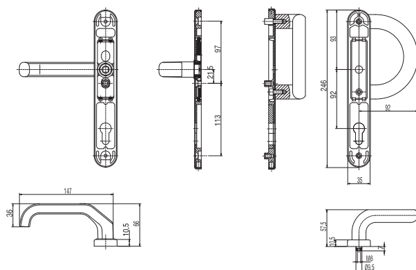
Klamka drzwiowa z pochwytem
