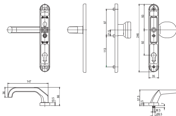
Klamka drzwiowa z gałką
