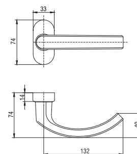
Klamka drzwiowa dzielona z szyldem owalnym
