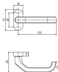
Klamka drzwiowa dzielona z szyldem owalnym
