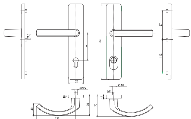
Klamka drzwiowa
