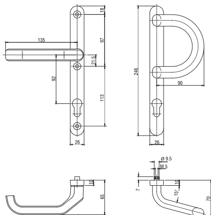
Klamka drzwiowa z pochwytem typu V
