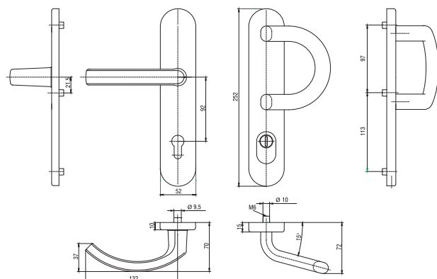
Klamka drzwiowa z pochwytem typu P
