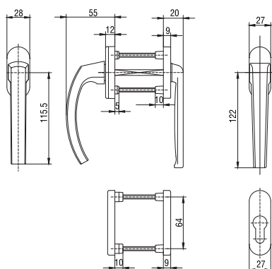
Komplet balkonowy pod żaluzję z szyldami owalnymi
