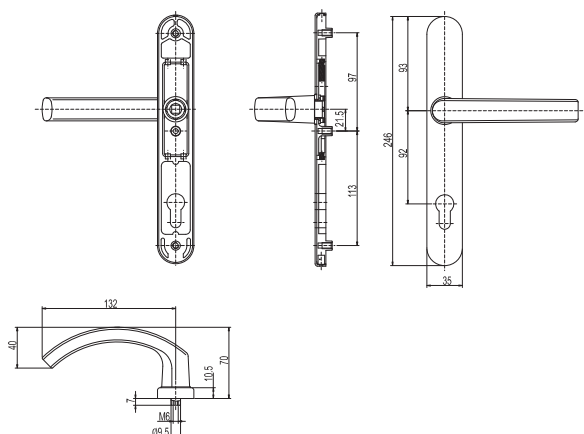
Klamka drzwiowa z pochwytem V
