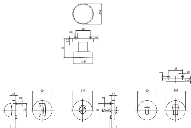
Obustronna gałka
