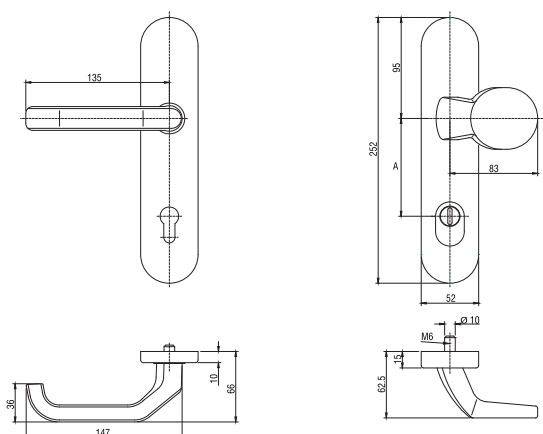
Klamka drzwiowa z gałką
