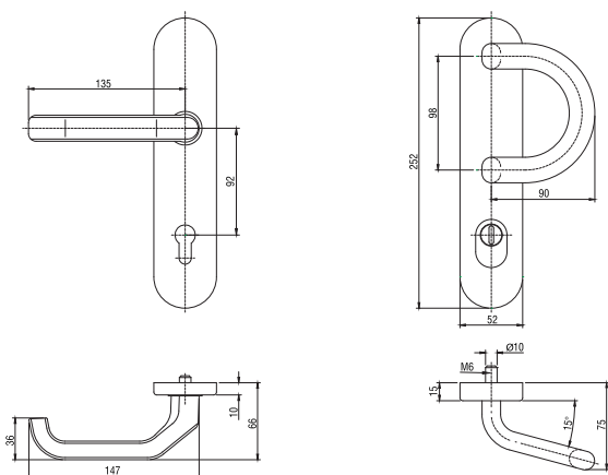
Klamka drzwiowa z pochwytem typu P
