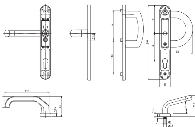
Klamka drzwiowa z pochwytem typu P
