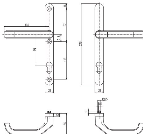
Klamka drzwiowa pod żaluzję
