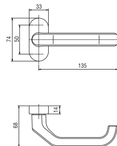
Klamka drzwiowa dzielona z szyldem owalnym
