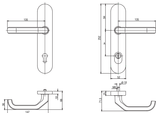
Klamka drzwiowa z pochwytem typu P
