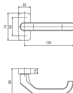
Klamka drzwiowa dzielona z szyldem prostokątnym
