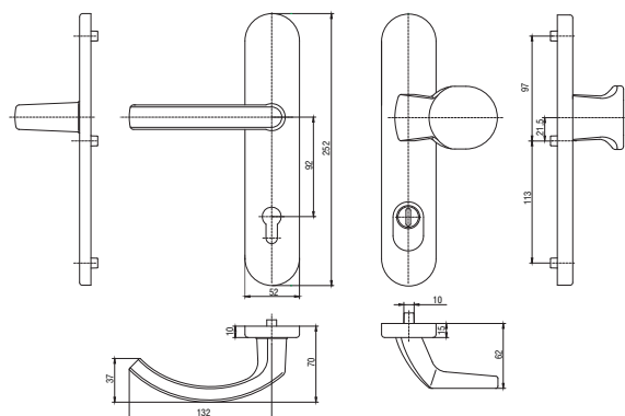
Klamka drzwiowa z gałką
