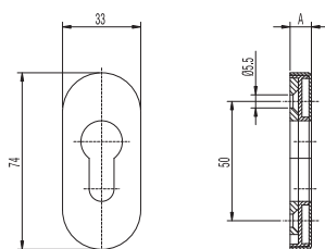
Szyld wkładki patentowej owalny
