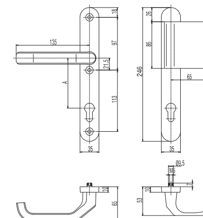
Klamka drzwiowa z pochwytem typu L
